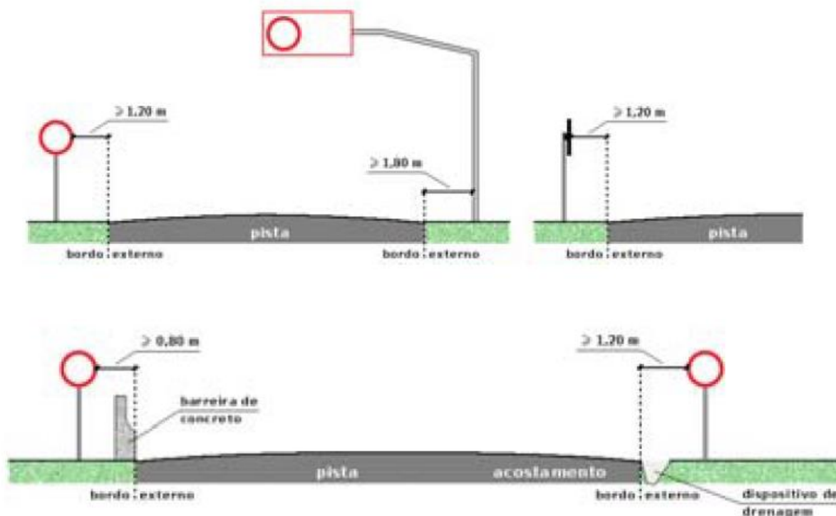
Figuras 1 e 2 – Instalações de placas de regulamentação em vias rurais
