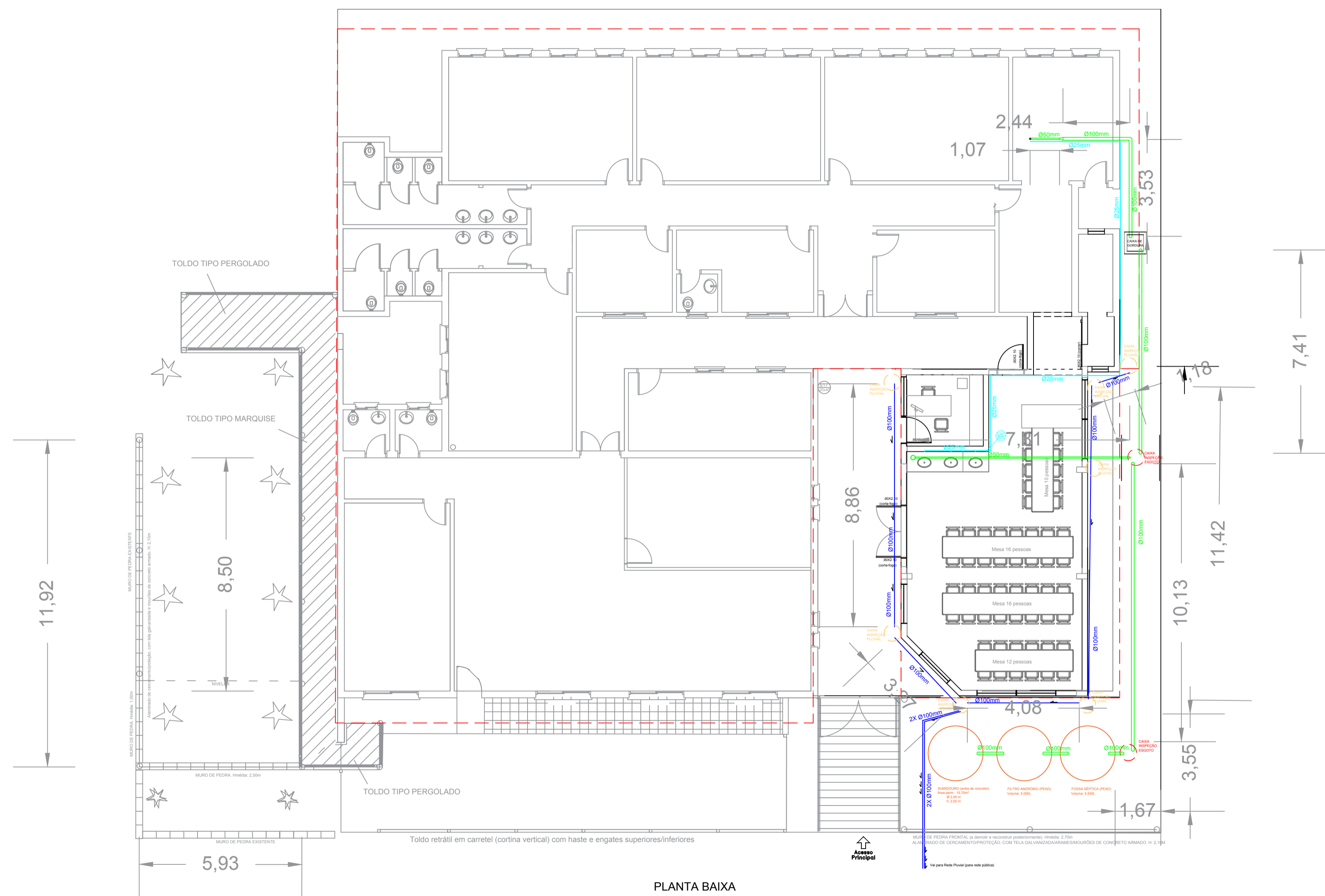
PLANTA BAIXA
