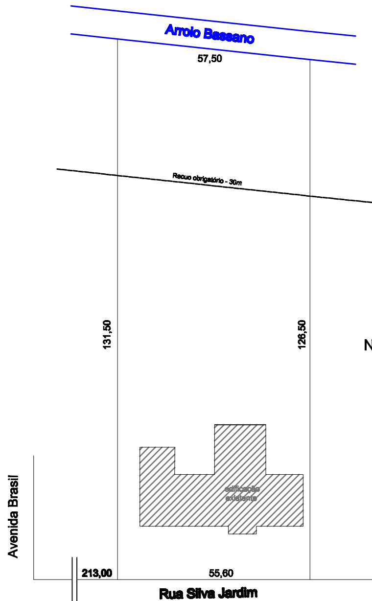
01. PLANTA DE SITUAÇÃO esc: 1/500
