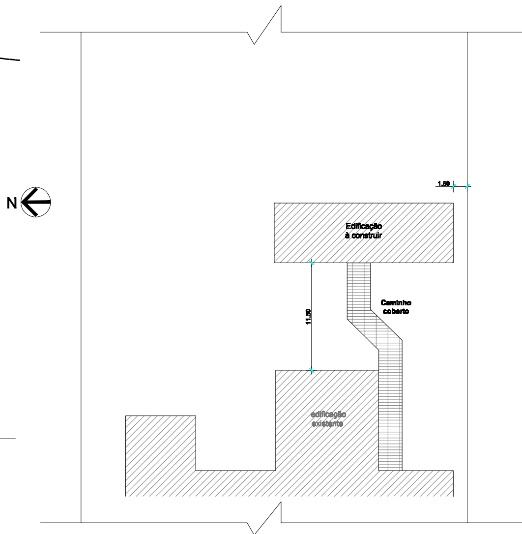
02. PLANTA DE LOCALIZAÇÃO esc: 1/200
